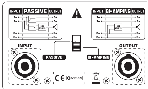
Рис. 1.2: Панель подключений сабвуфера (B1800X PRO)
